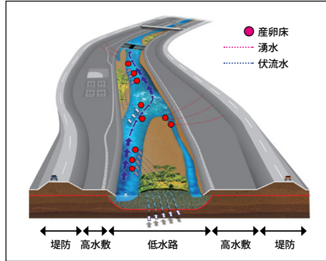
イラスト 豊平川の模式図（再掲） Aruga et al. (2023) Environ Biol Fish 一部改変（→p6）
