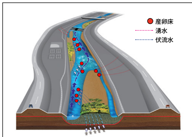
イラスト 豊平川の模式図 Aruga et al. (2023) Environ Biol Fish 一部改変
